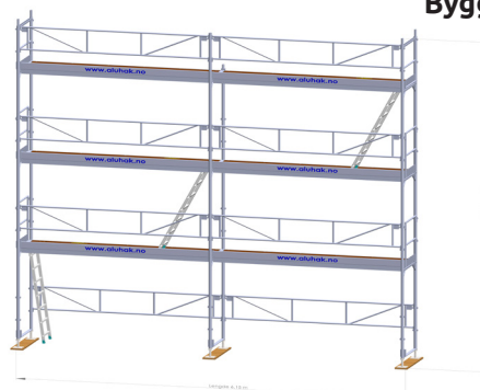
Byggemåte B-2
